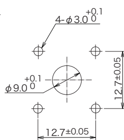
取付参考寸法
