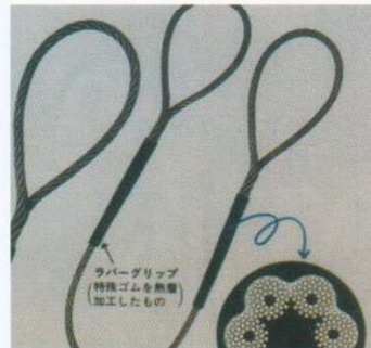
鋼索の結束 (NPR)
