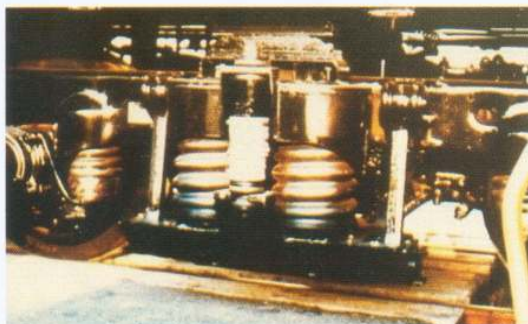
車輪用スプリングの防雪カバー (SPC)
