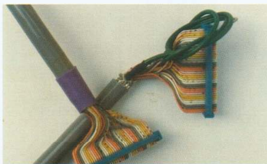
インターフェイスケーブルのコネクター接続部 (NPE)
